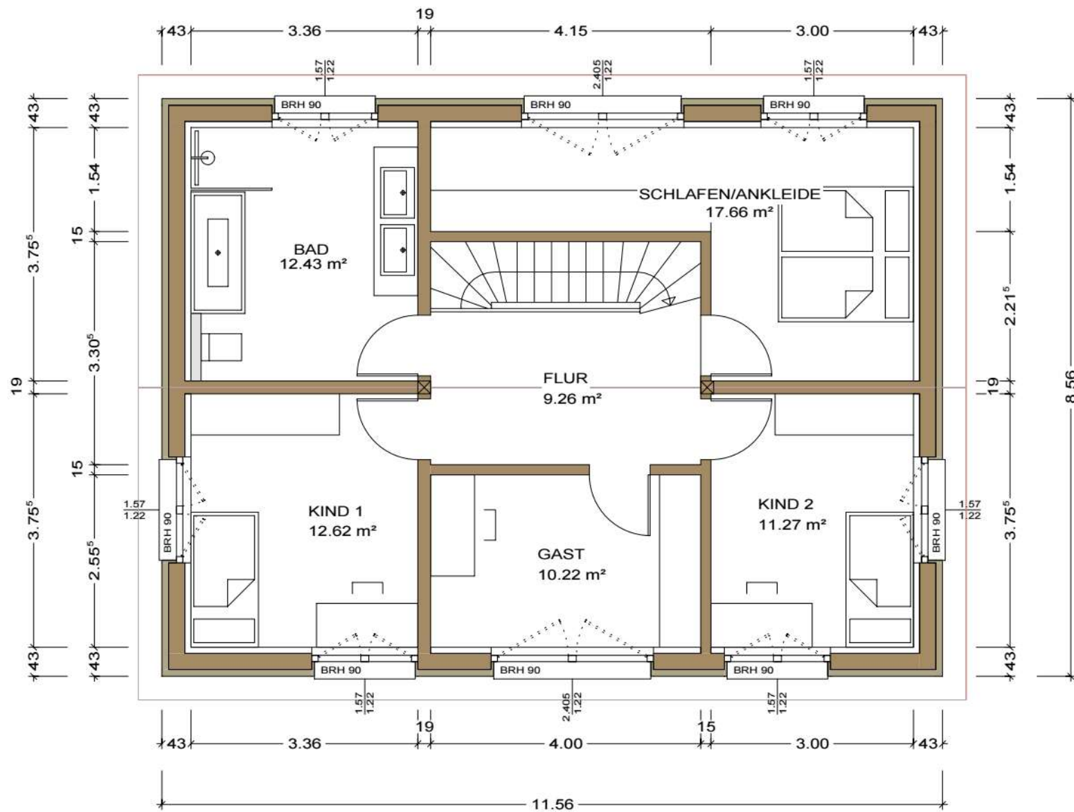
GRUNDRISS OBERGESCHOSS
