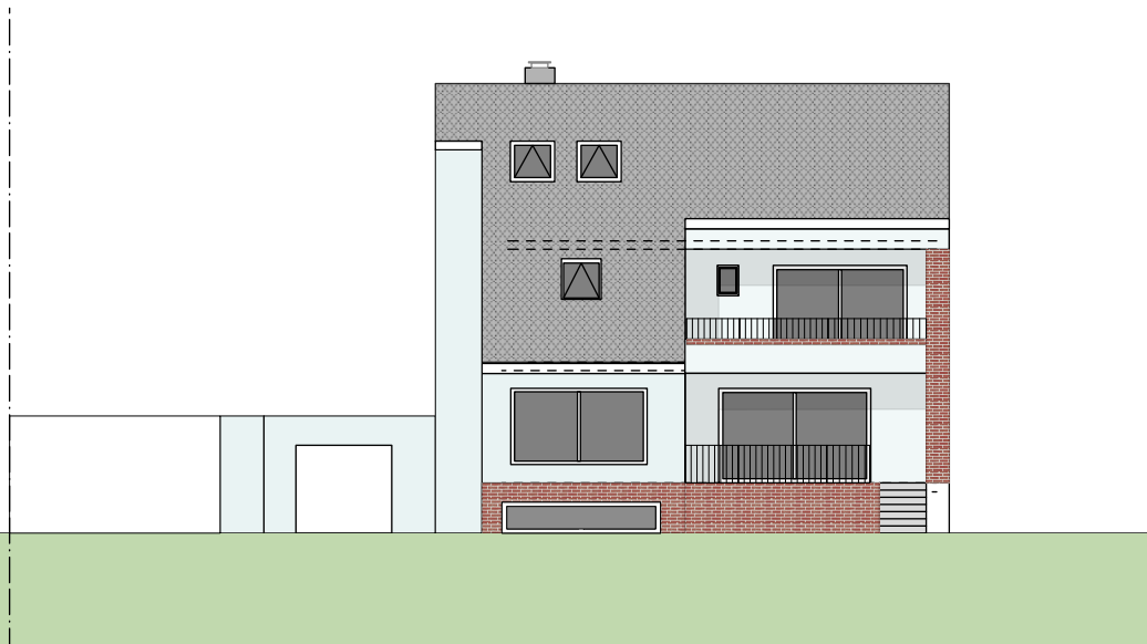
Ansicht Westen
