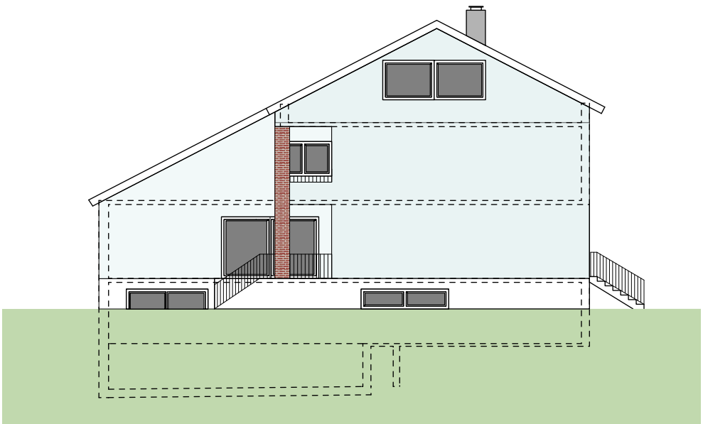
Ansicht Süden
