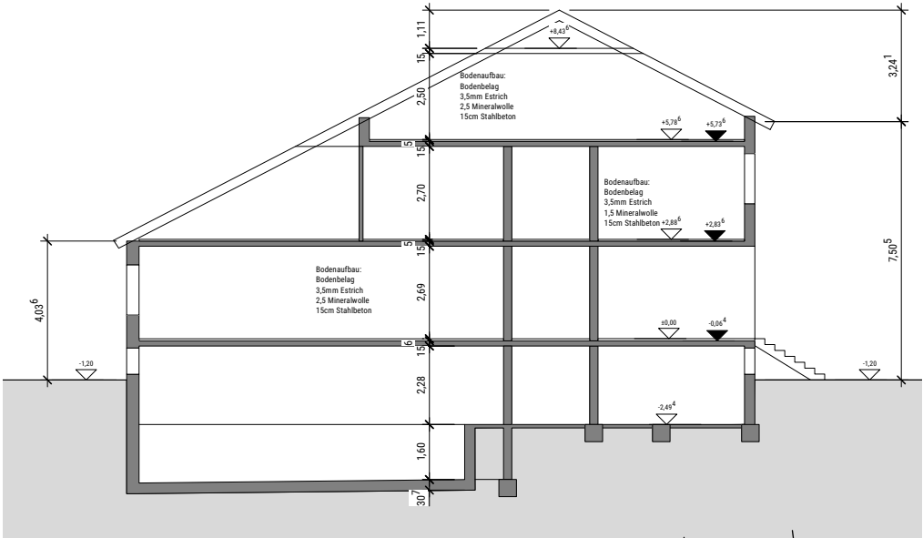
Schnitt
