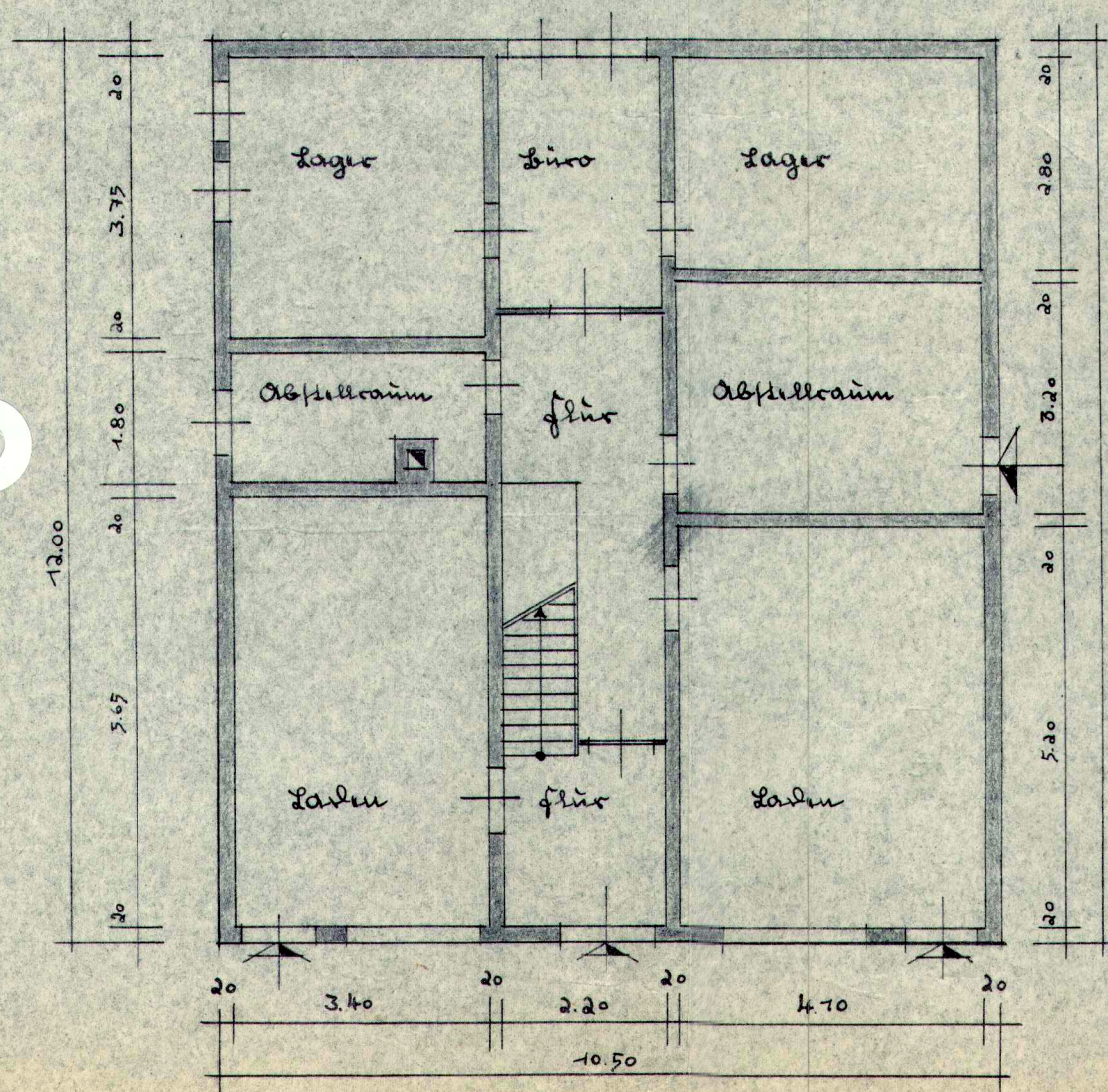
Grundriss
