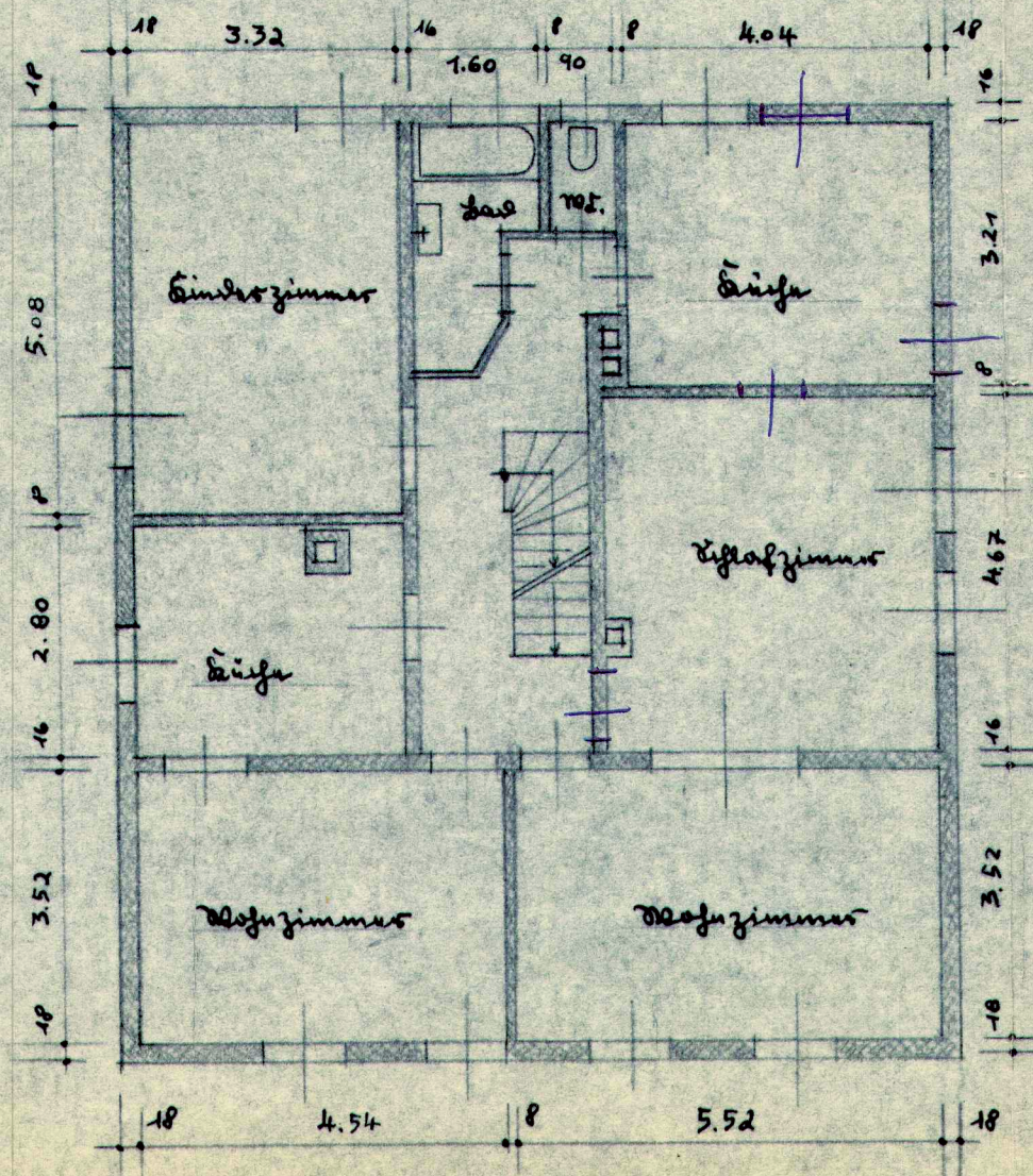
Obergeschossgrundriß
