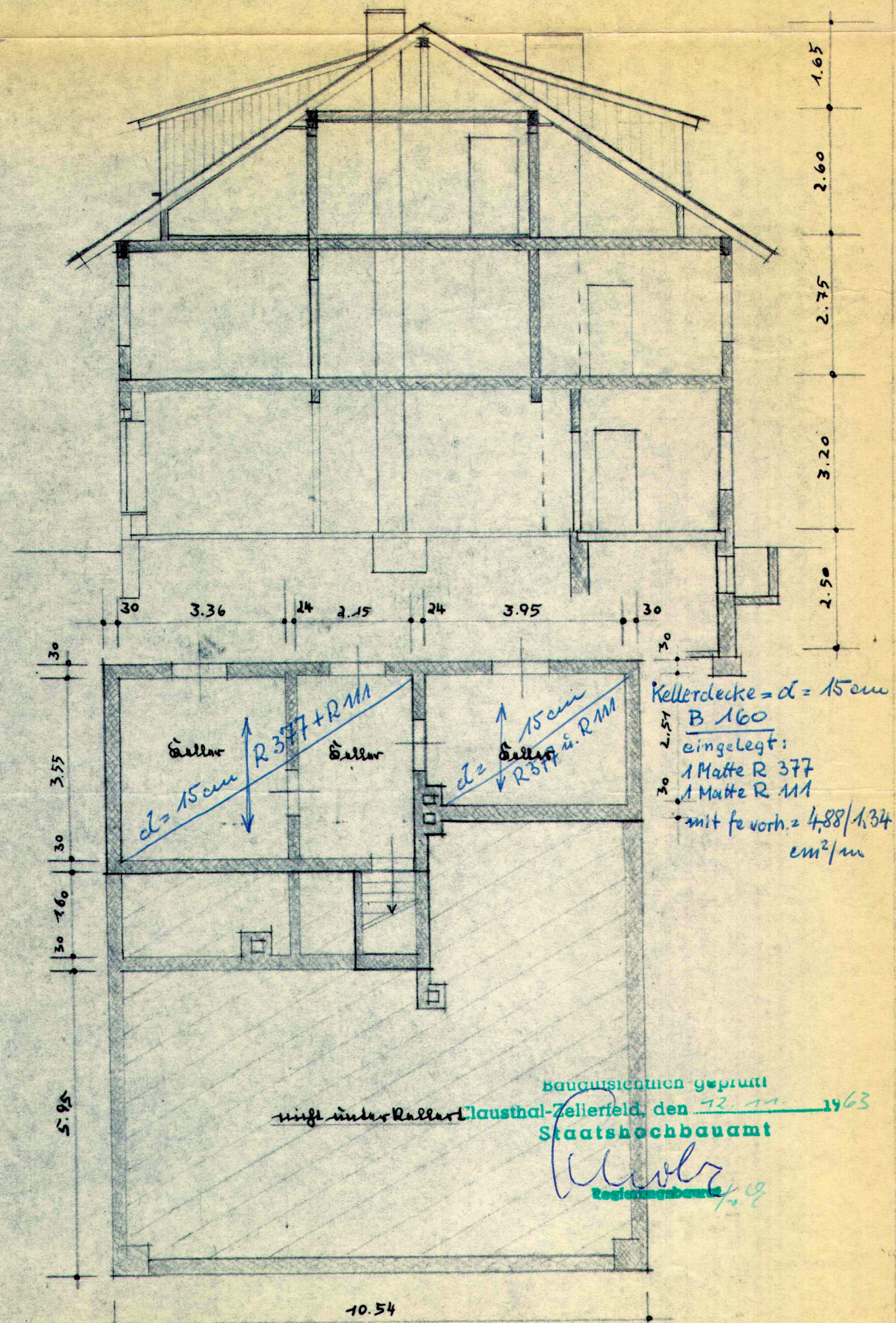
Querschnitt
