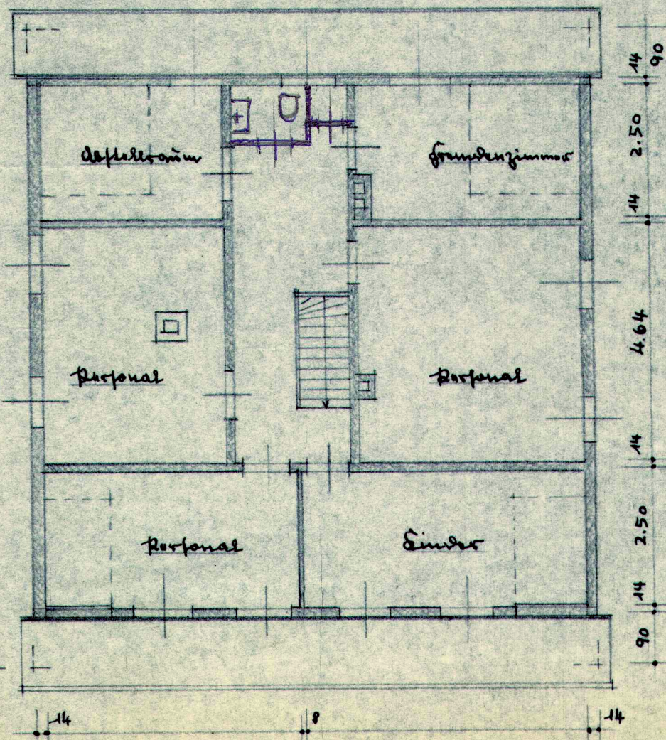
Vorhangsfassgrundriß
