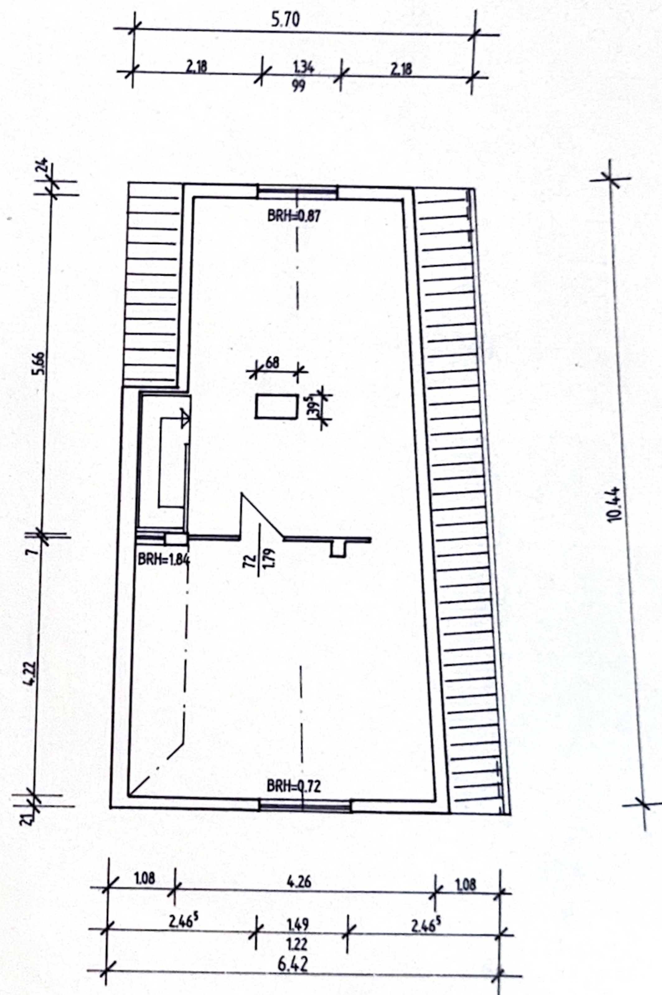
DACHGESCHOSS
