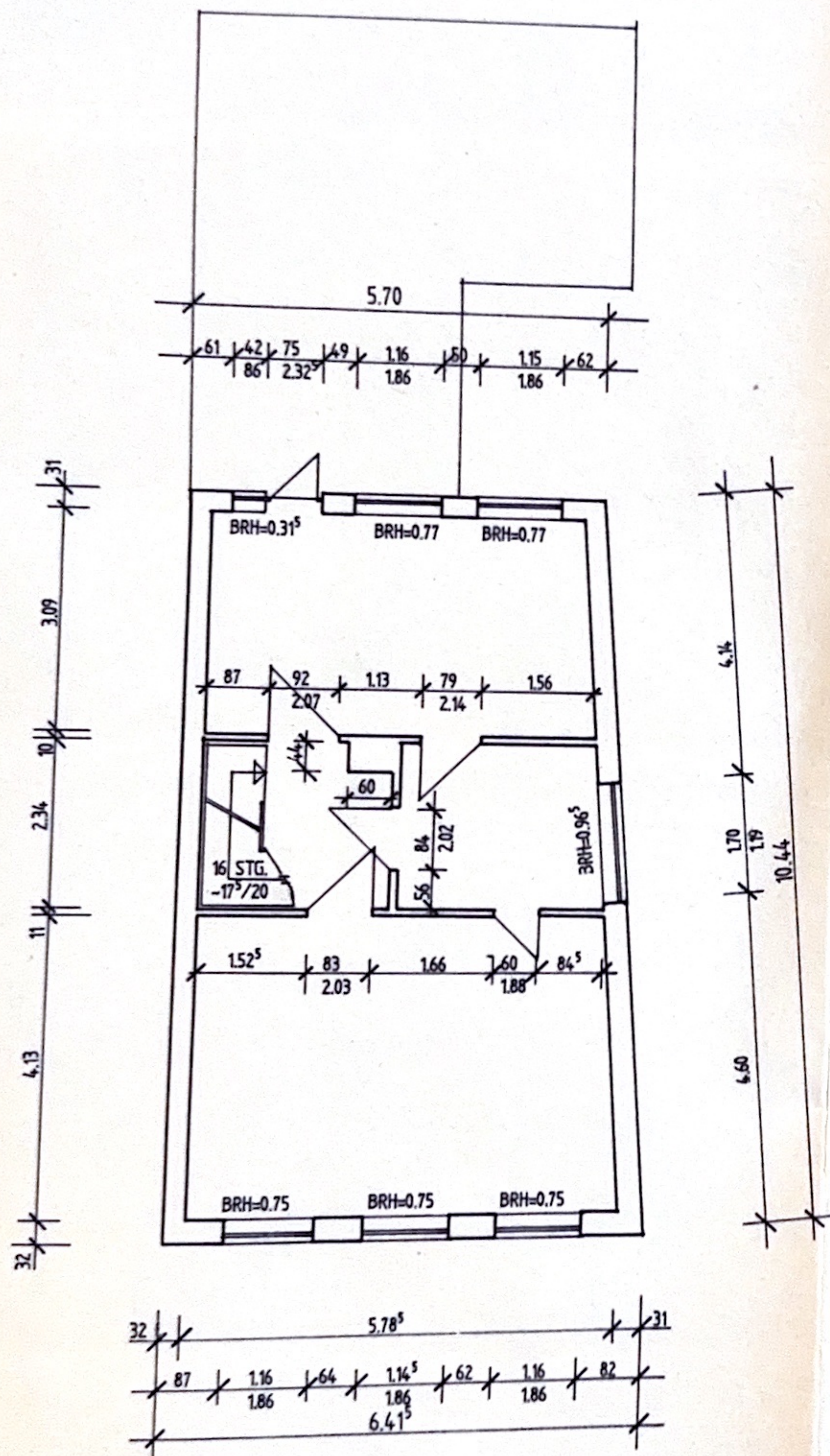
OBERGESCHOSS
