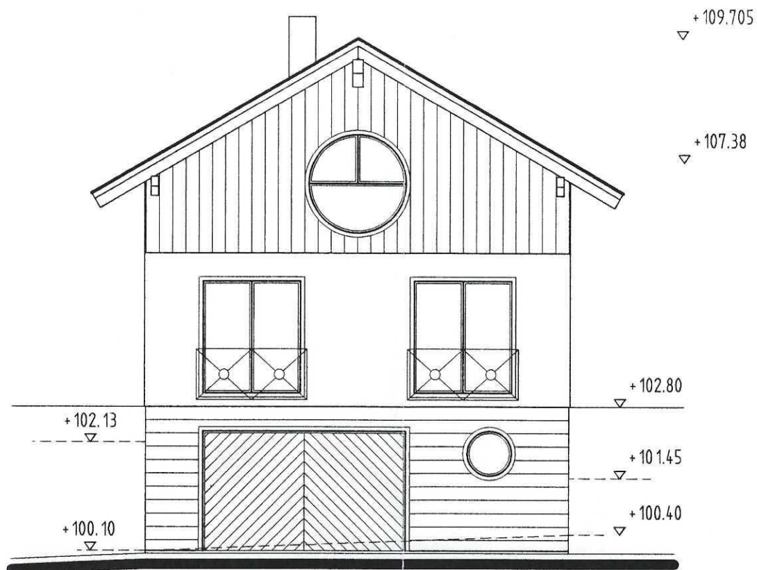
SÜD - ANSICHT
