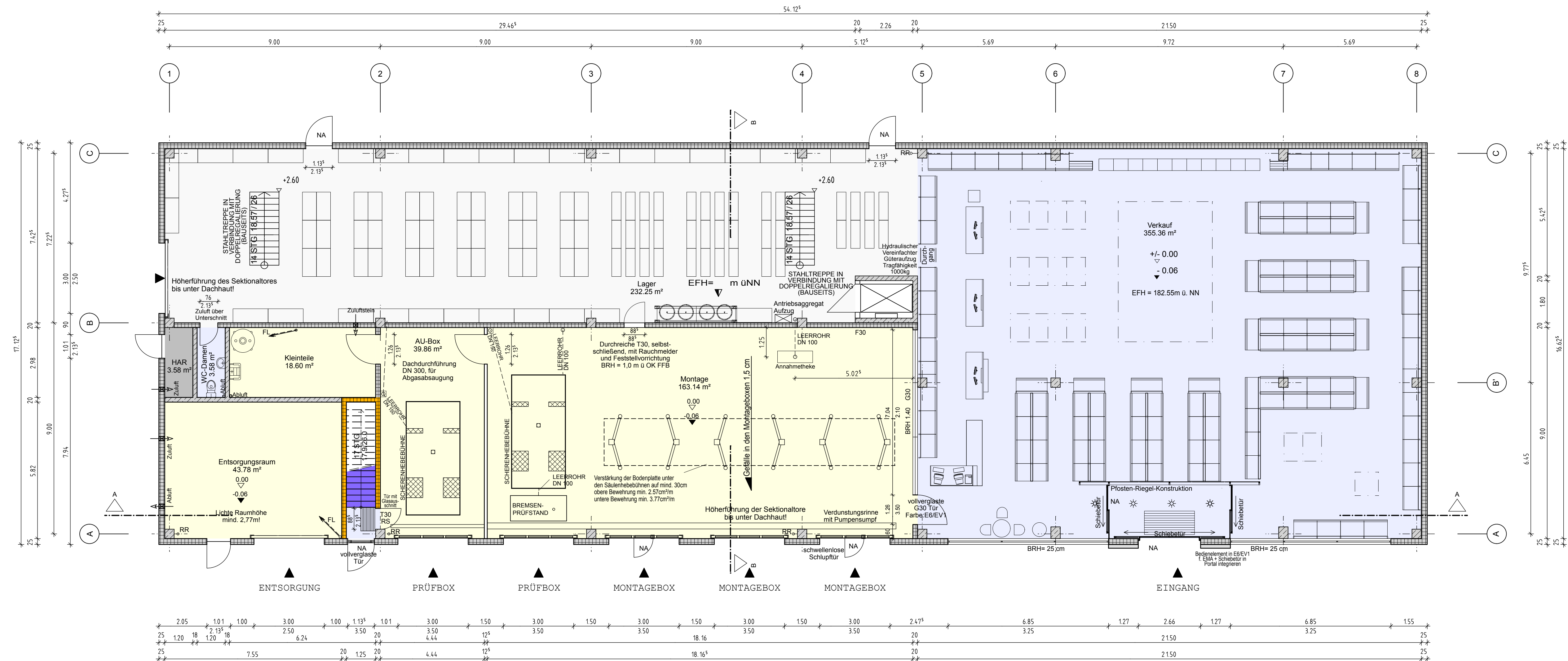
Grundriss EG M. 1/100
