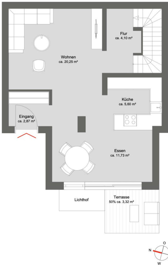
Grundriss Erdgeschoss
